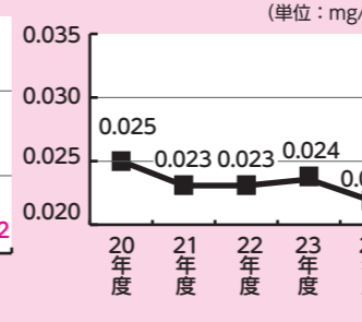
■浮遊粒子状物質濃度の経年変化(年平均値)
